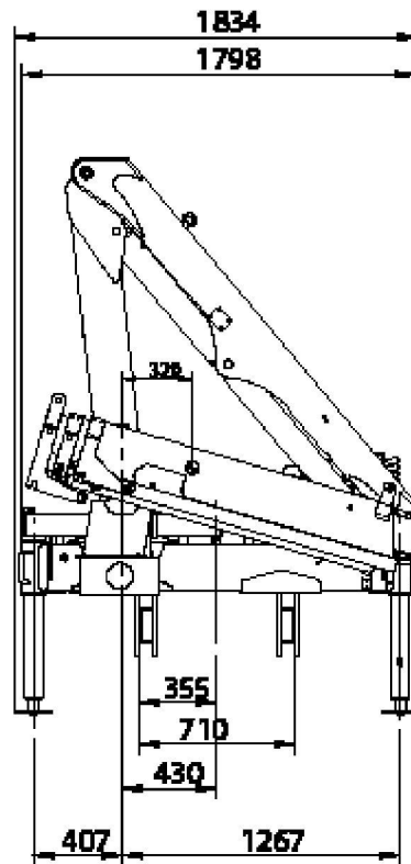
Ingombri versione R Dimensions R version
